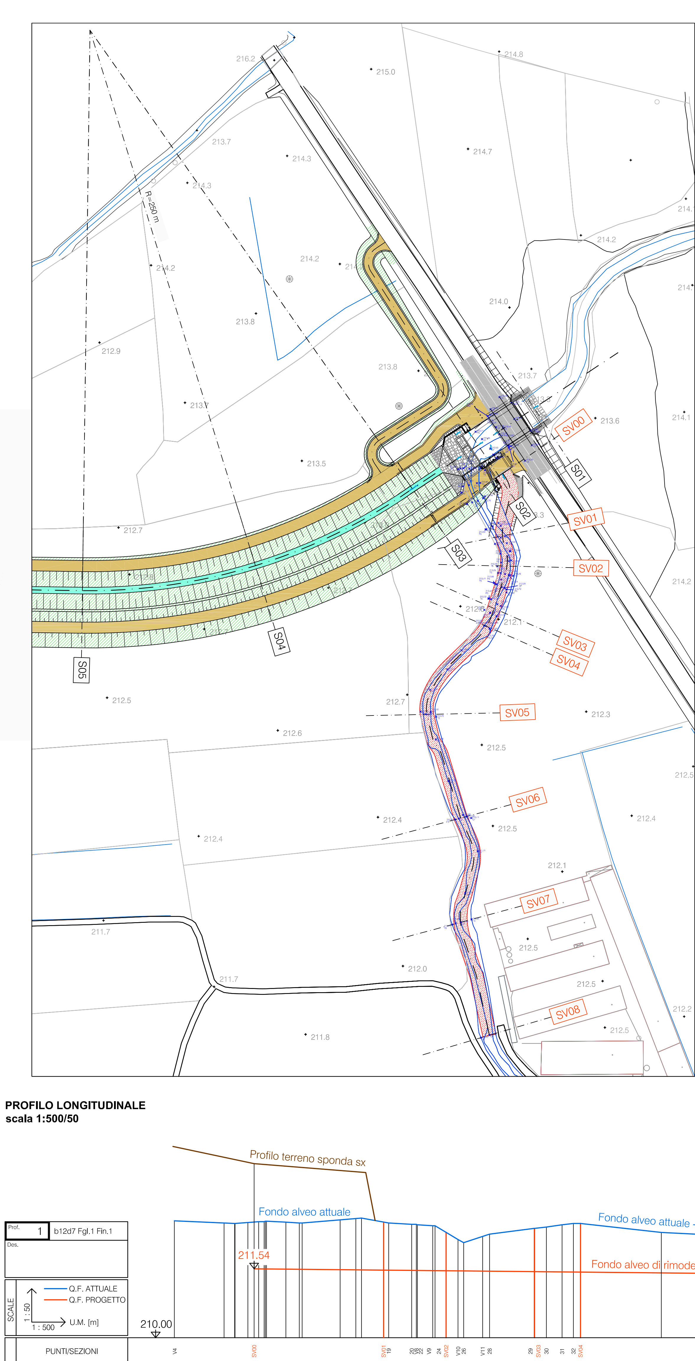
PROFILLO LONGITUDINALE scala 1:500/50
